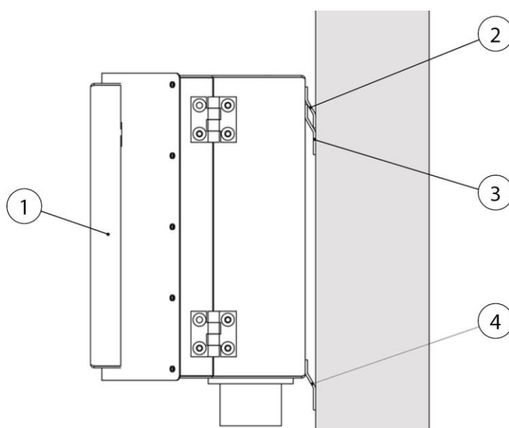
Fig. 8: Montering av styringsboks
