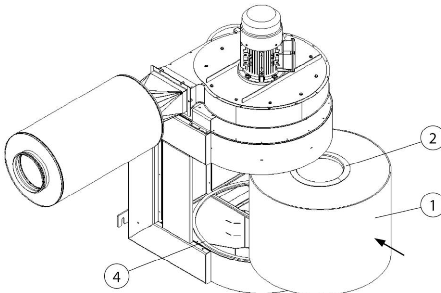
Fig. 15: filterbytte
